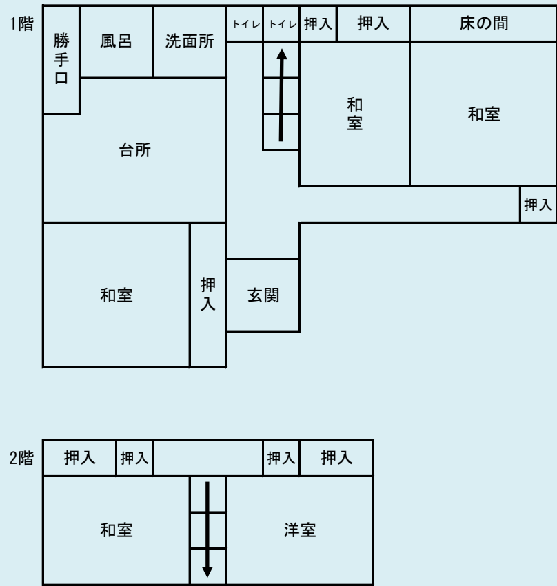
間取り（概況）
